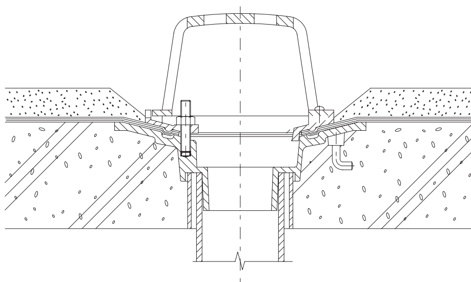
施工例:RJ-AB
