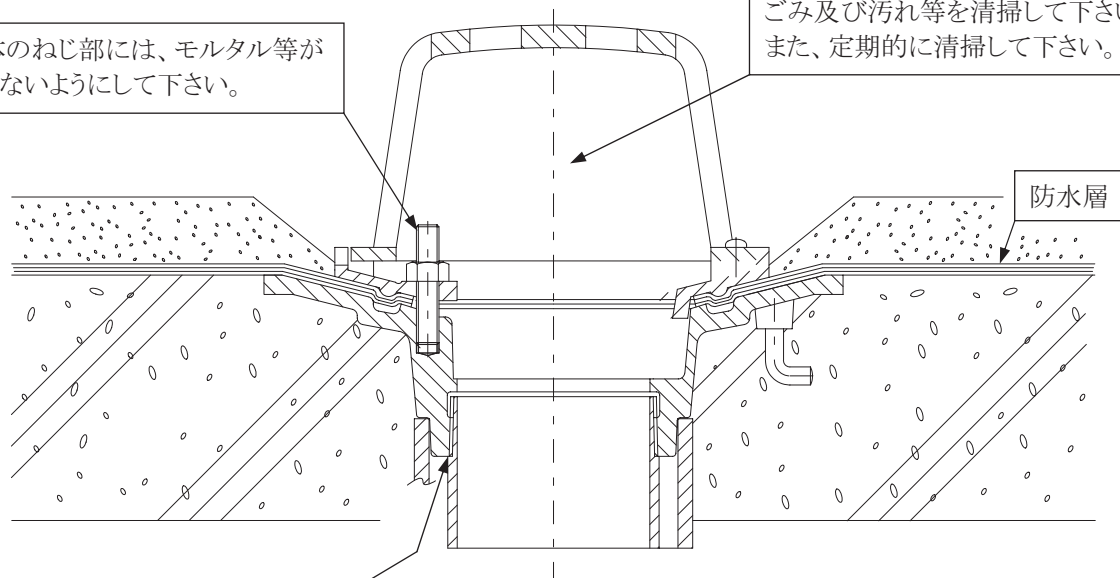
施工例:RJ-AA
