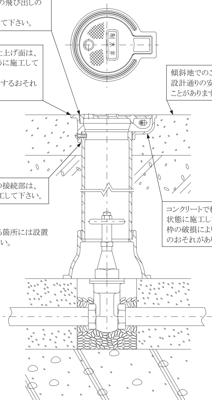
施工例:B5
