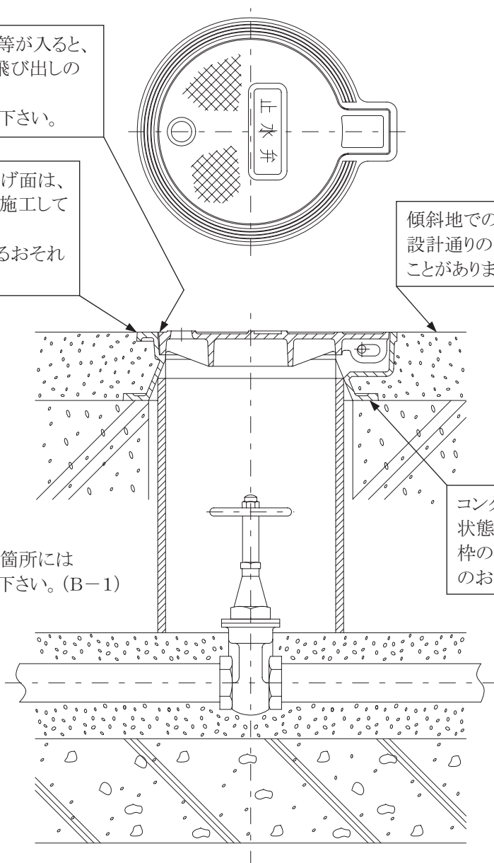
施工例:B-1
