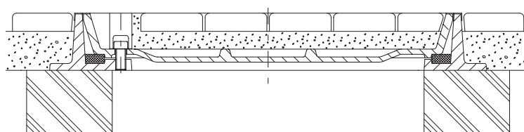
施工例：密閉形（ボルト・パッキン式）
