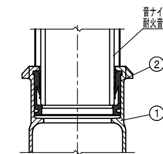
上部立て管接続部詳細
