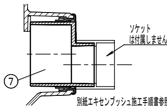
エキセンブッシュ接続部詳細
