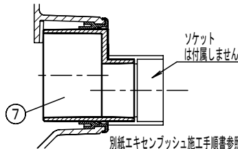
別紙エキセンブッシュ施工手順書参照 エキセンブッシュ接続部詳細
