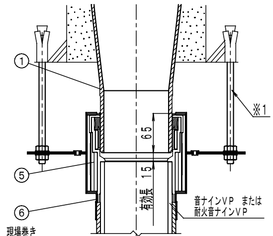
下部立て管接続部詳細
