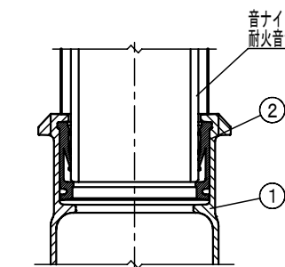
上部立て管接続部詳細
