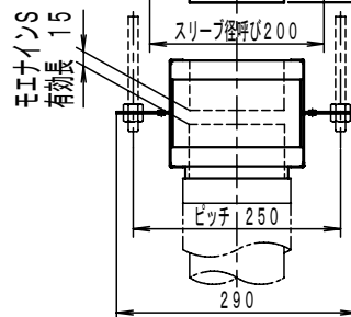
エキセンブッシュ接続部詳細
