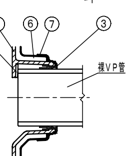
横枝管接続部詳細
