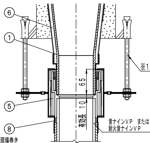
下部立て管接続部詳細
