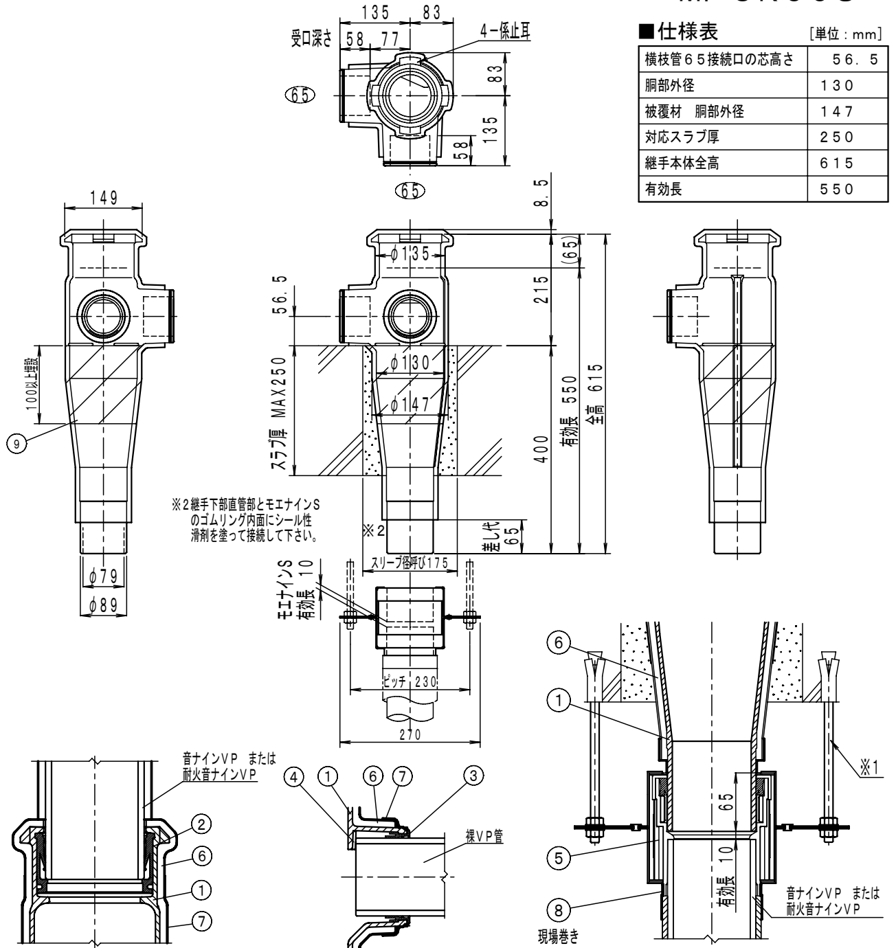
上部立て管接続部詳細
