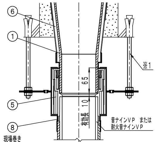
下部立て管接続部詳細
