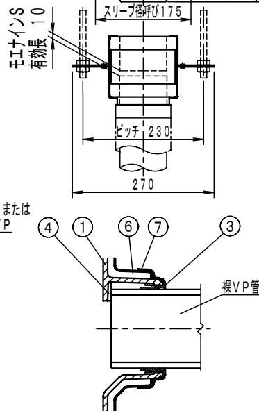
横枝管接続部詳細
