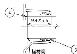
横枝管接続部形状
