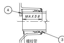
横枝管接続部形状
