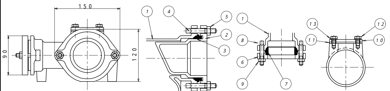
三角ふた装着部形状
