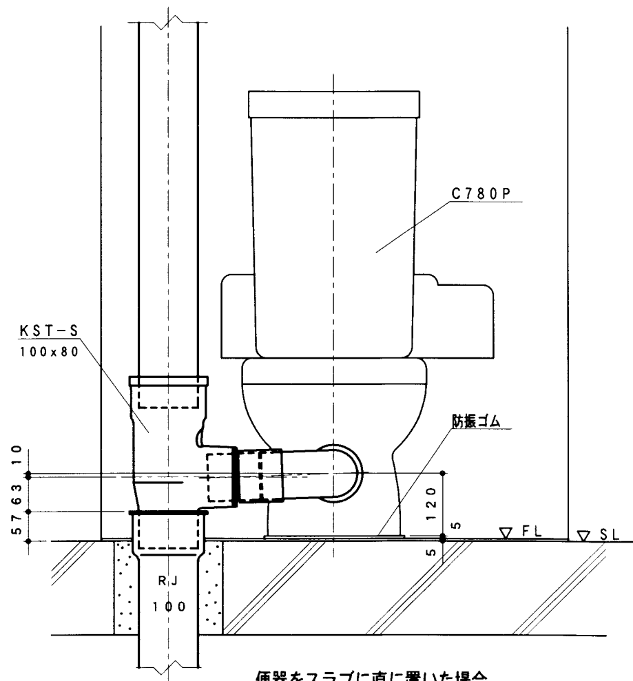
KST-S 100x80 と RJ100 を接続する場合の配管例
