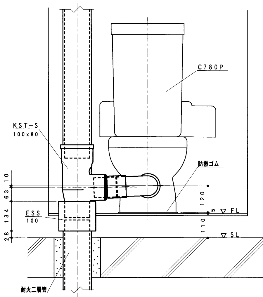
KST-S 100x80 と ESS100 を接続する場合の配管例
