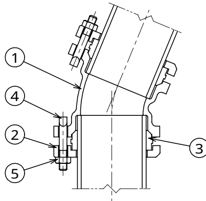
立て管接続部形状
