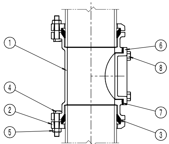
Y-Y線断面図
