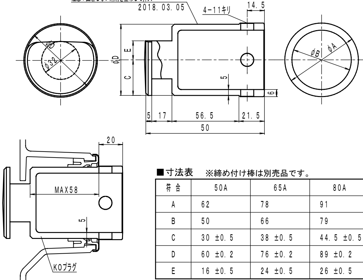
KOプラグ接続部形状
